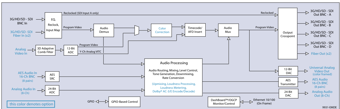
9931-EMDE 9931-EMDE Block Diagram
